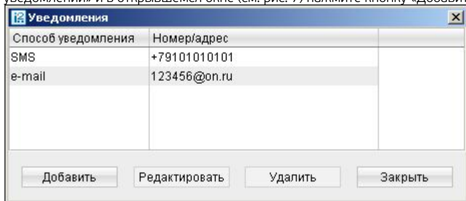
Рис. 7. Уведомления
