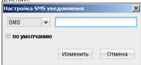
Рис. 8. Добавление уведомления
