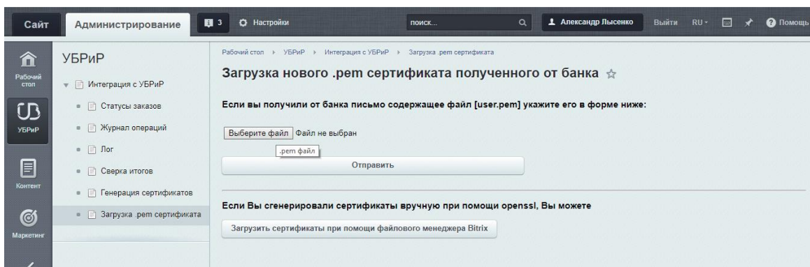
Рисунок 5. Загрузка сертификата
