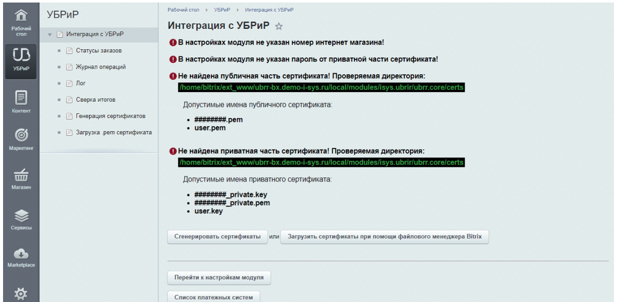
Рисунок 2. Настройка модуля
