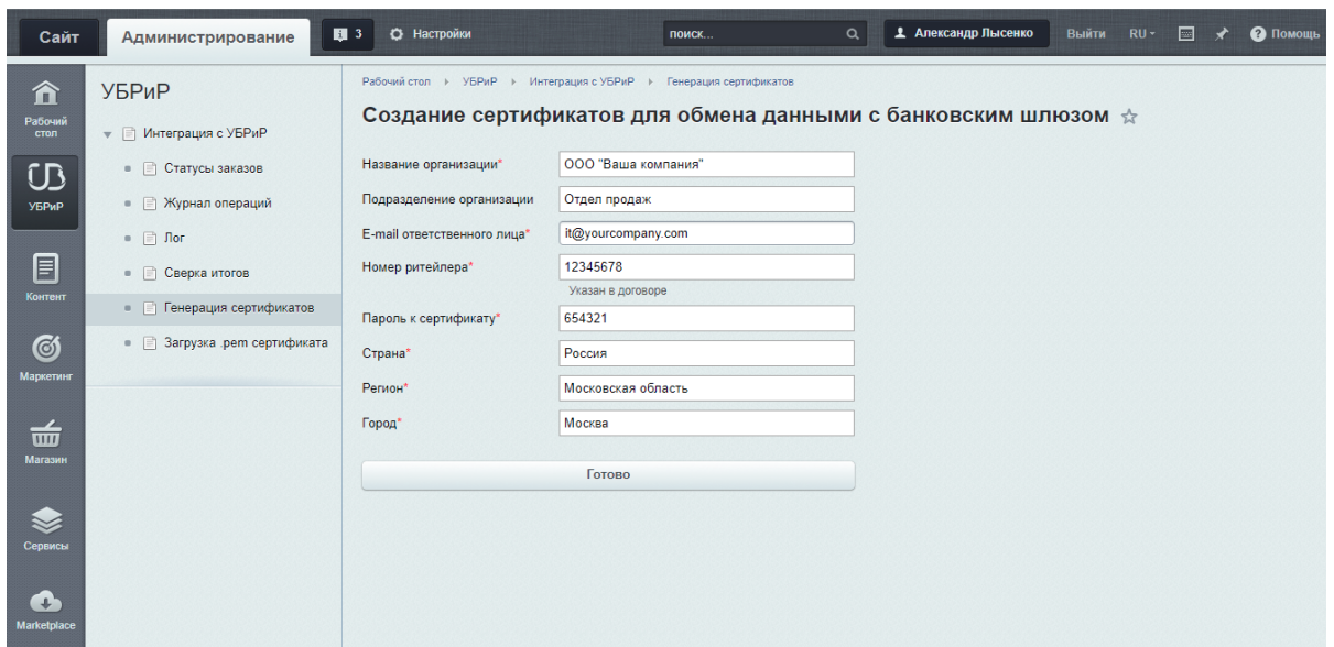
Рисунок 3. Генерация сертификатов
