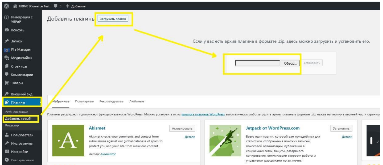
Рисунок 3. Установка плагина
